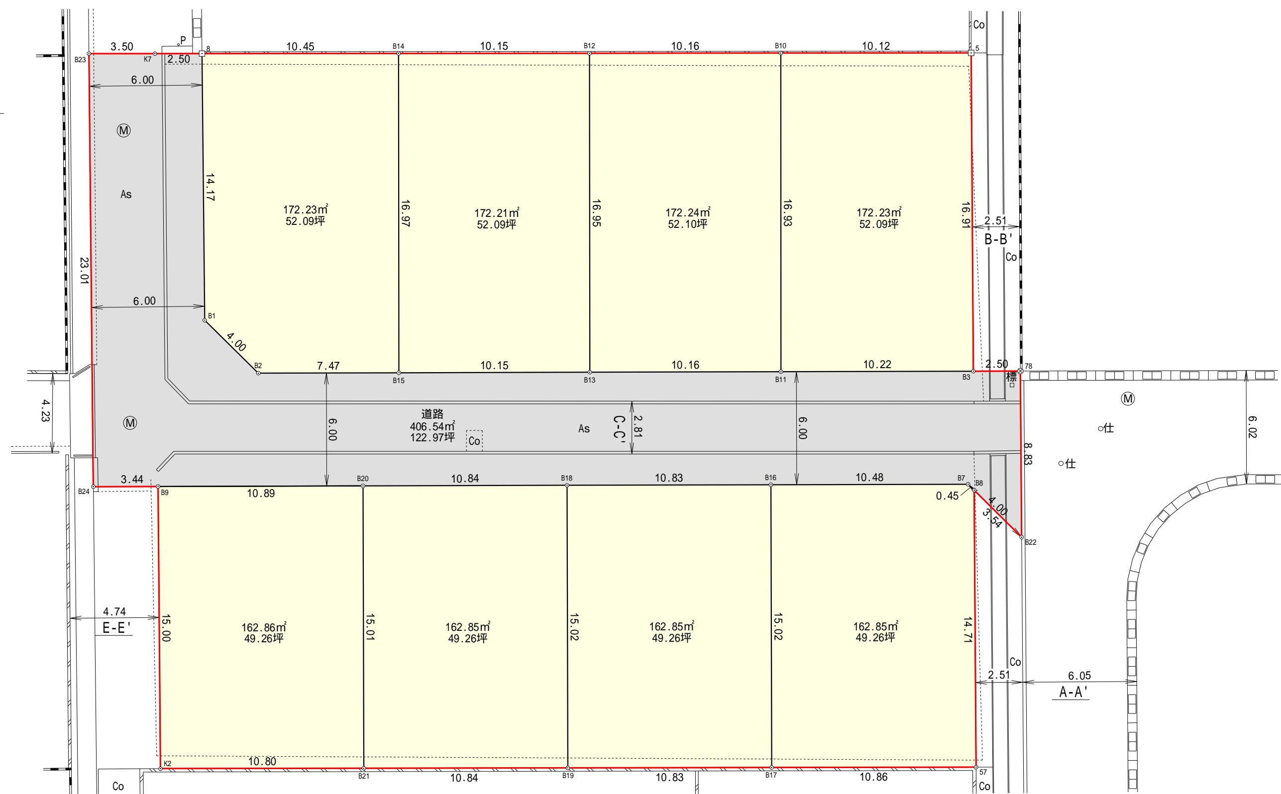
土地利用計画表
